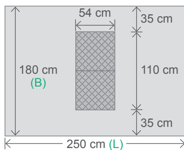
3: Fiberdugen lægges ud i bunden af udgravningen på underlag og perforeres i bunden. Placer BIO-BLOK® elementerne med lodret stående rør. Undgå så vidt muligt jord m.m. på duget.
